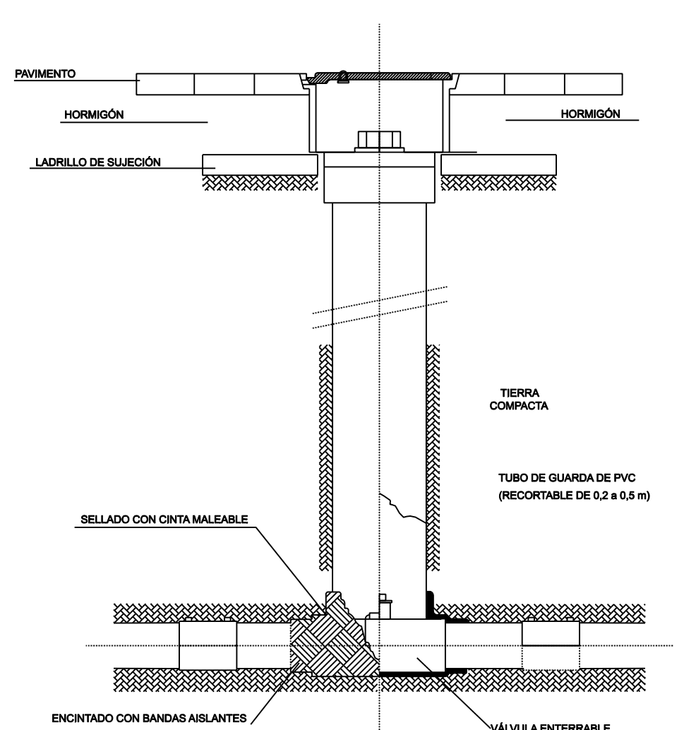
CONJUNTO DE MONTAJE TAPA Y MARCO DE FUNDICIÓN
